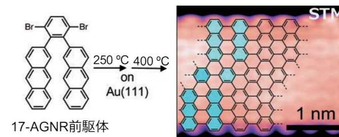
図3 前駆体から金基板上で合成した17-AGNRのSTM分子イメージ。17は幅方向の炭素原子の数。 17-AGNR: \Delta E_g = 0.2 \text{ eV} on Au(111)
