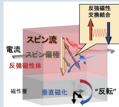
反強磁性体中で生成されたスピル流を使った、隣接磁性層の磁化反転の様子
