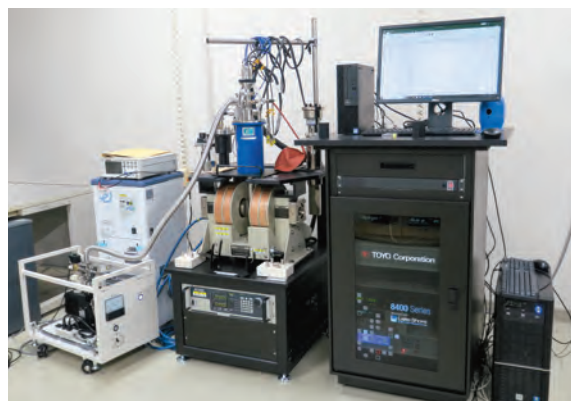
ホール測定システム
