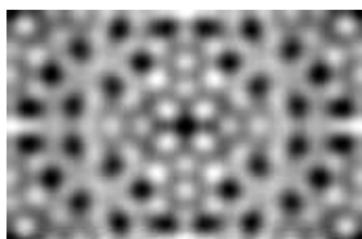
塩素置換したフタロシアニン銅薄膜結晶の円環視野像と分子構造
