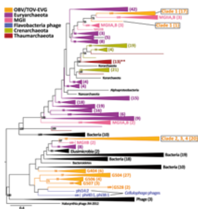
海洋メタゲノムから発見されたグループII 海洋古細菌ウイルスの分子系統樹
